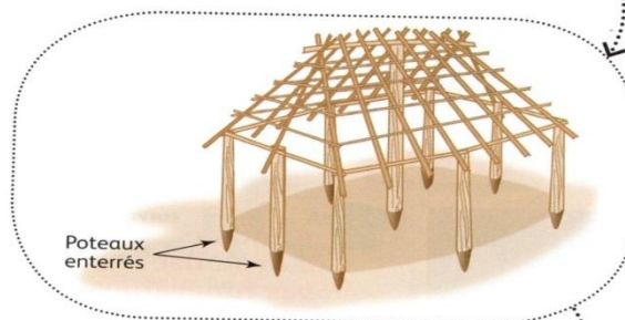
b. Dessin fondé sur un relevé de traces archéologiques
